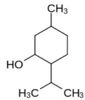
Pfefferminz -> Menthol
