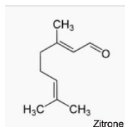
Zitrone
