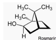
Rosmarin
