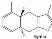
Myrrhe
