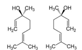
Salbei
