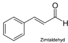
Zimtaldehyd
