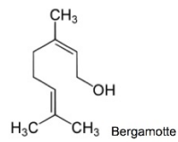
Bergamotte
